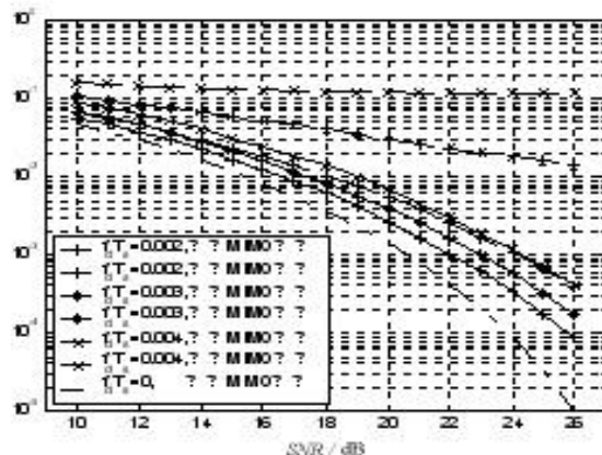
(b) 自举均衡系统与常规均衡系统误码性能比较(L=256)
