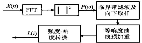
图2 BSD方法的听觉转换模型
