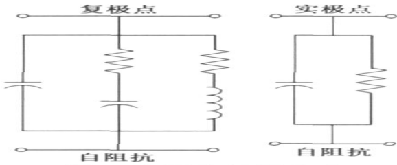
图 2 自阻抗等效电路
