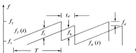
图1 线性调频连续波的发射和接收波形
