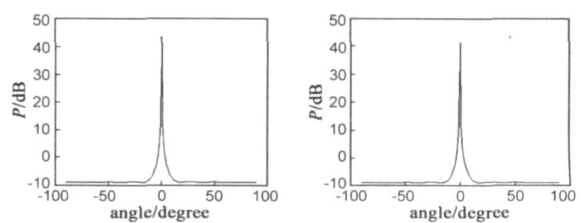
(a) 协方差为 1 时, 模拟目标的 MUSIC 谱图 (b) 协方差为 11 时, 模拟目标的 MUSIC 谱图
