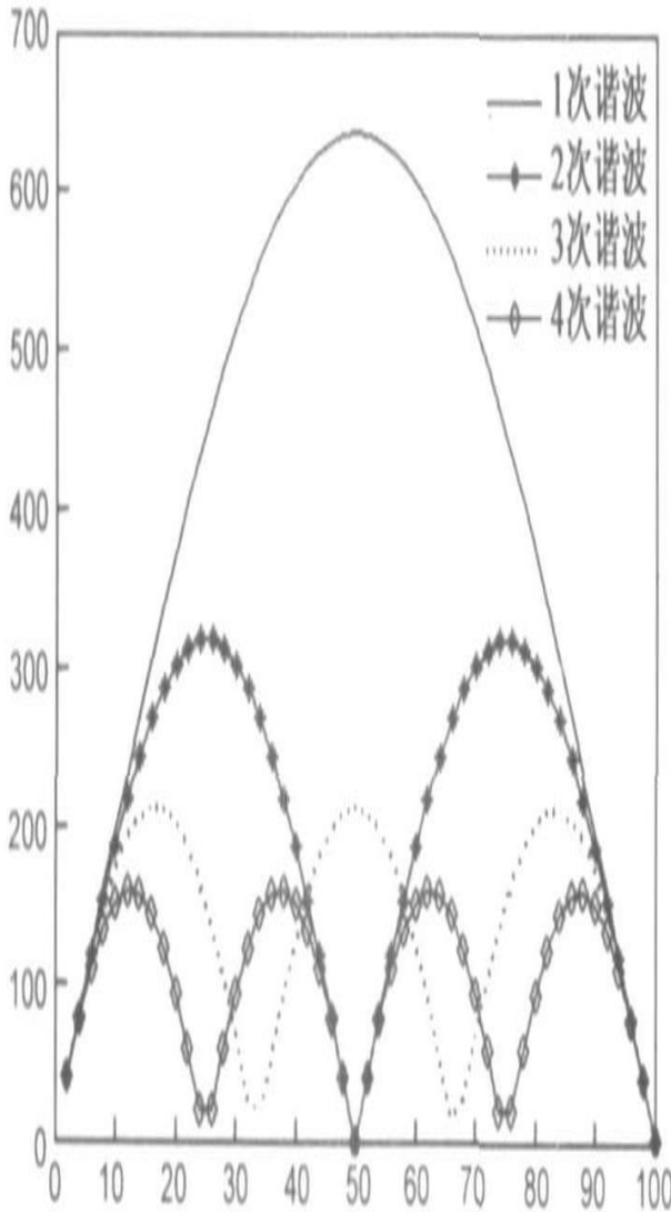
图3 占空比与脉冲谐波能量分布关系
