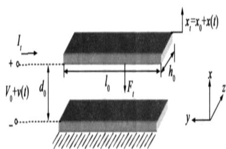
图1 静电换能器示意图
