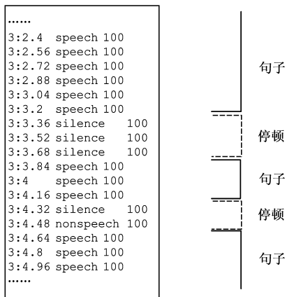
图2 音频片段分类结果
