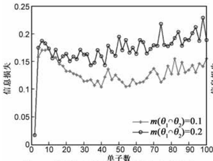
图4 冲突焦点低赋值随单子个数增加对信息损失的影响
