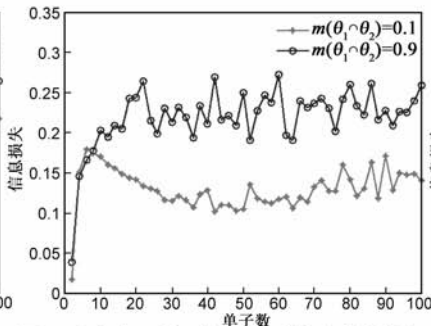
图5 冲突焦点高、低赋值随单子个数增加对信息损失的影响
