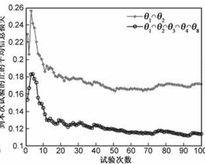
图2 信息损失与冲突焦点之间的关系
