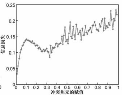
图3 冲突焦点赋值变化对信息损失的影响
