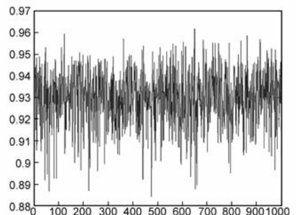
图9 融合结果的相似度
