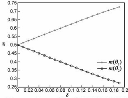
图7 m(\theta_1) 和 m(\theta_2) 随着 \delta 的增长的变化情况
