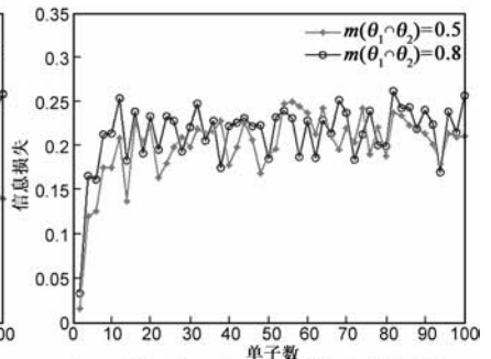
图6 冲突焦点高赋值随单子个数增加对信息损失的影响
