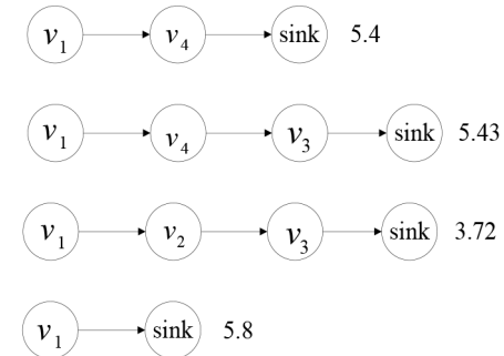
(b) v_1 到 sink 的所有可能路径
