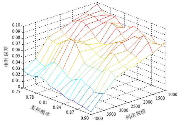
图11 算法精度分析
