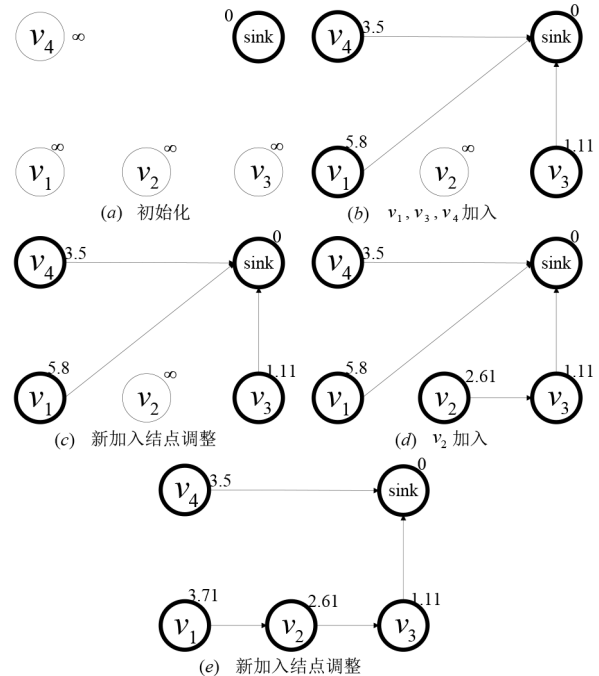
图3 算法的执行过程
