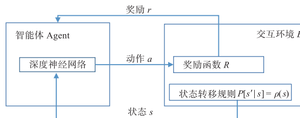
图1 深度强化学习框架
