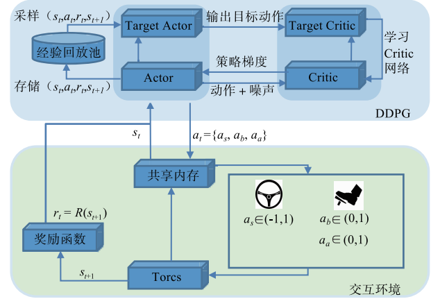
图2 系统模型
