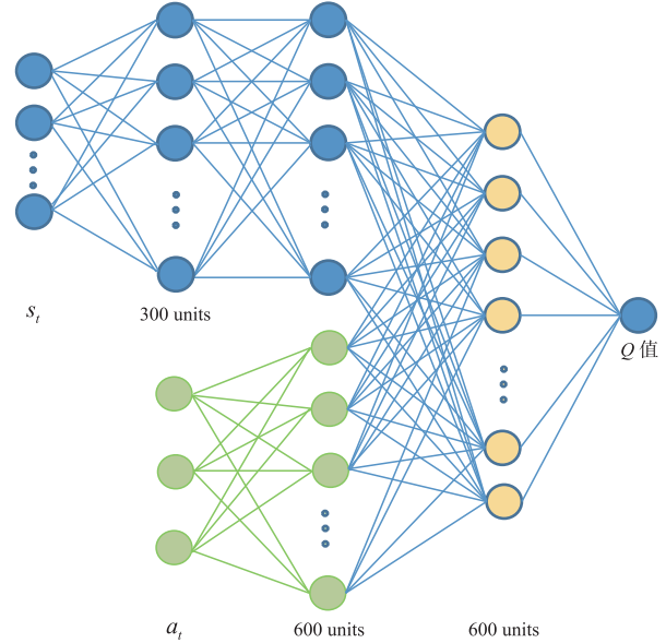
图5 Critic网络
