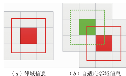
图1 邻域(3×3)信息的改进示意图
