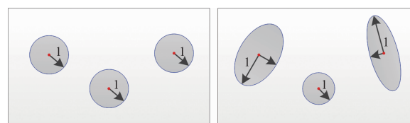
图3 欧式距离与马氏距离的差异
