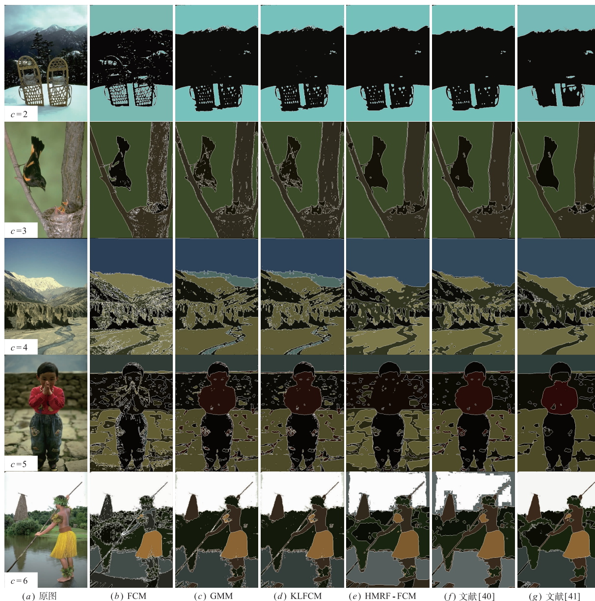
图14 六种算法对自然图像的分割结果
