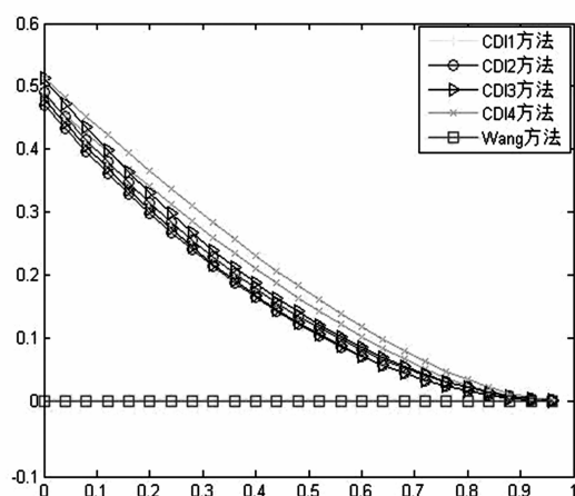
图1 m(A) 随 \varepsilon 的变化趋势图
