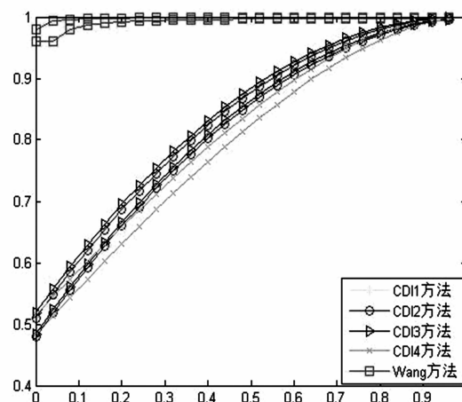
图2 m(B) 随 \varepsilon 的变化趋势图
