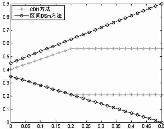
图3 焦元A的区间信度赋值随 \eta 变化趋势图
