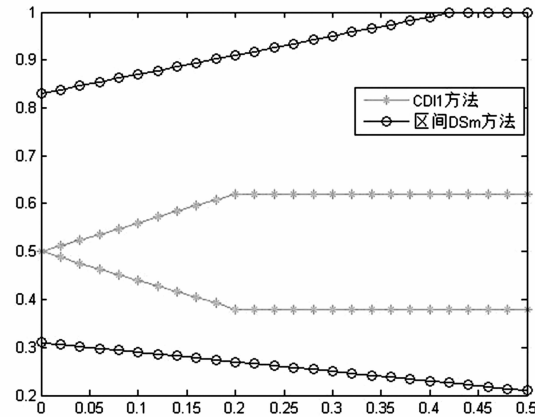
图4 焦元 A \cap B 的区间信度赋值随 \eta 变化趋势图
